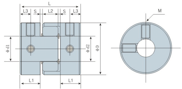
LK20-14~LK20-30
